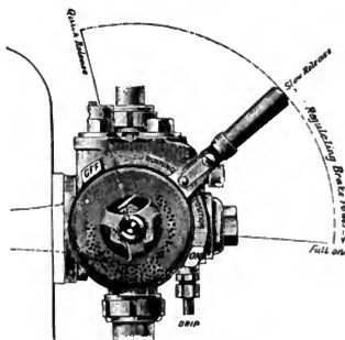
Fig. 5127. Locomotive Ejector.
